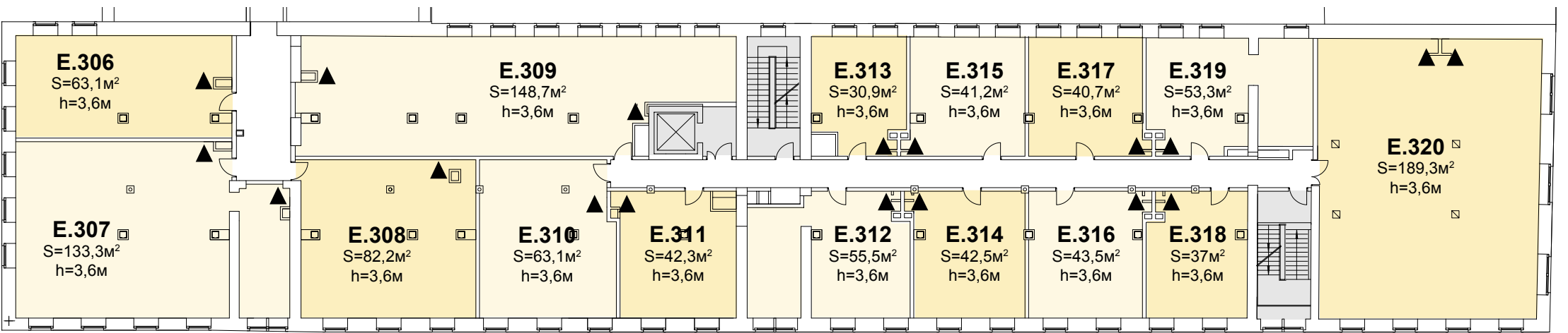
План 3-го этажа
