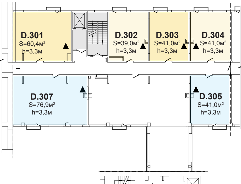
План 3-го этажа
