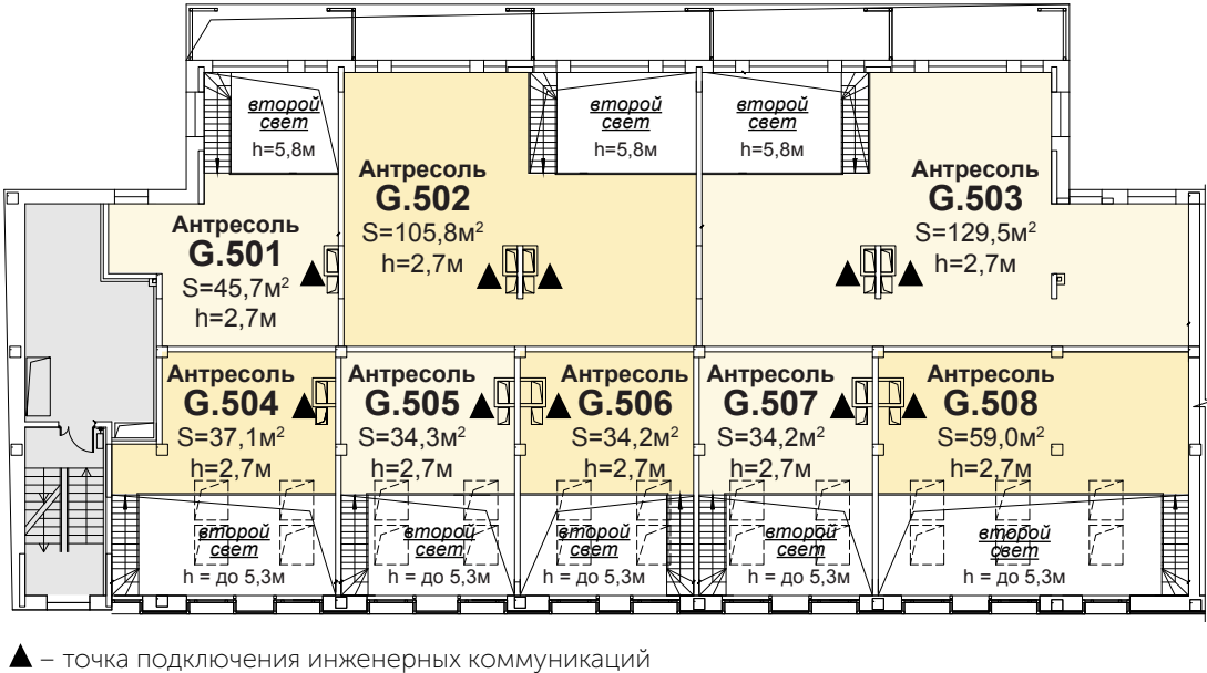
План антресоли 5-го этажа
