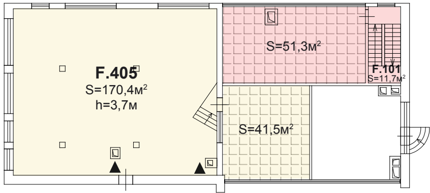
План 4-го этажа
