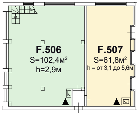
План 5-го этажа
