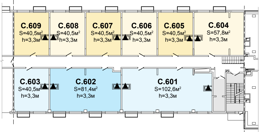
План 6-го этажа
