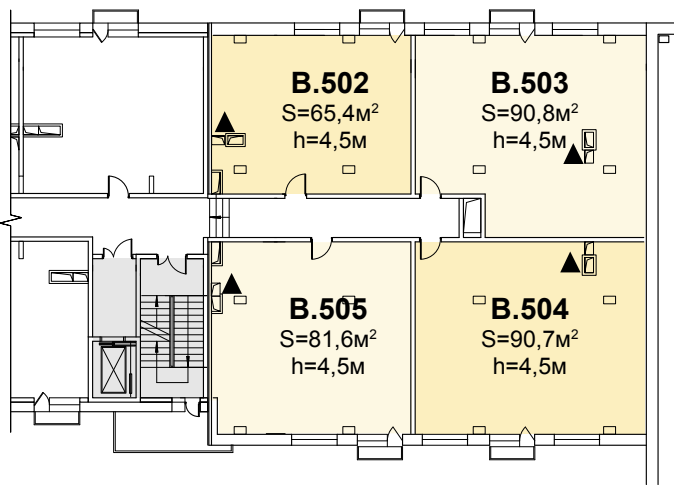
План 5-го этажа
